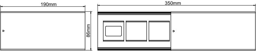
STS-SC03 3 modules unit
