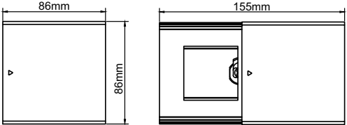
STS-SC03 1 modules unit
